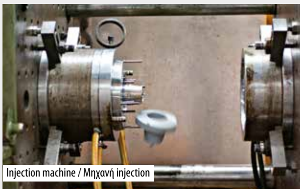
Injection machine producing globe pre-form Μηχανή injection παράγει pre-form μπάλας
